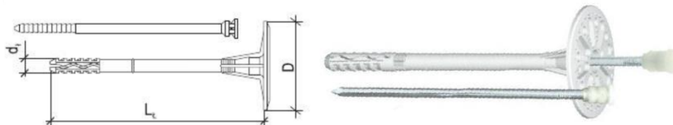
Дюбел за изолация с метален пирон LMX
